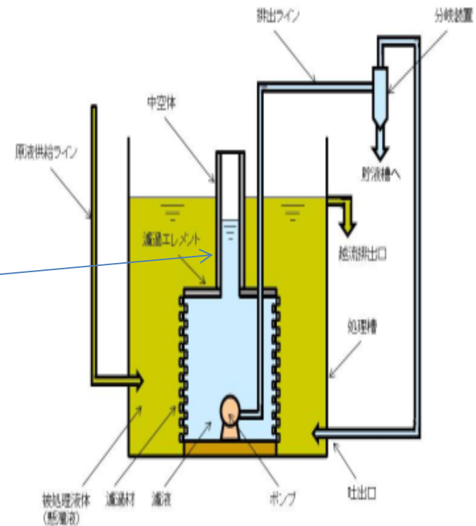
図-1 液体処理装置の構成
