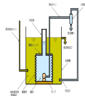
図-1 液体処理装置の構成
