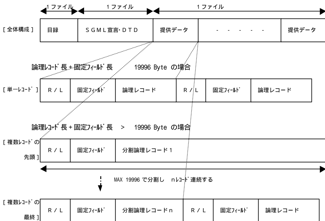
図 3.3.2 提供データファイルのレコード構成
