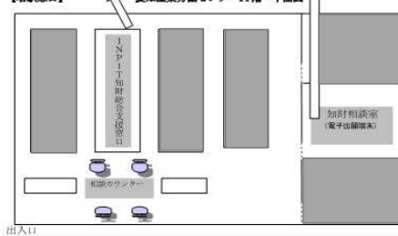
【栄・伏見窓口】執務スペース 詳細図
